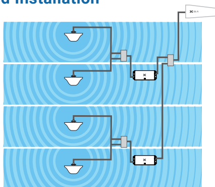
4 Omni Antennas
